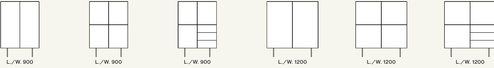
Box Modulo H. 1104 x P./D. 478 - 542
